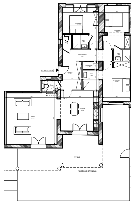
Echelle 1/200°
